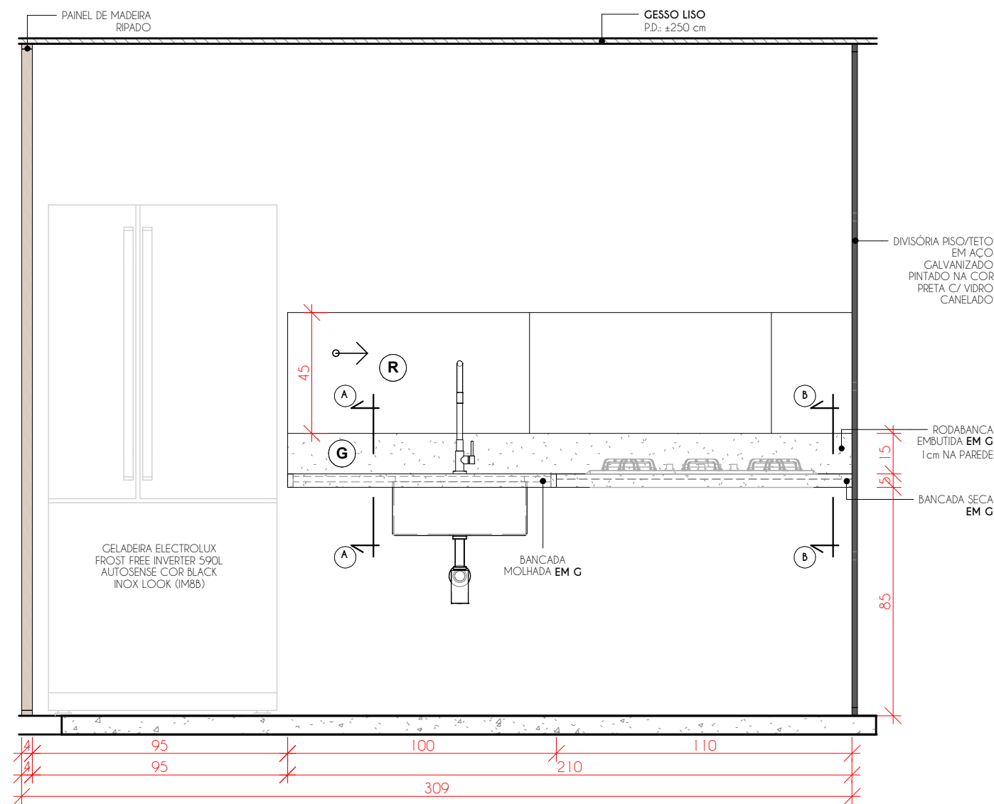
VISTA B ESCALA 1 : 20
